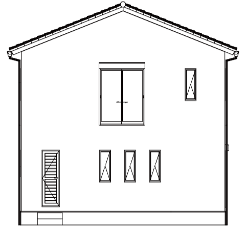
西側 立面図 S:1/100
