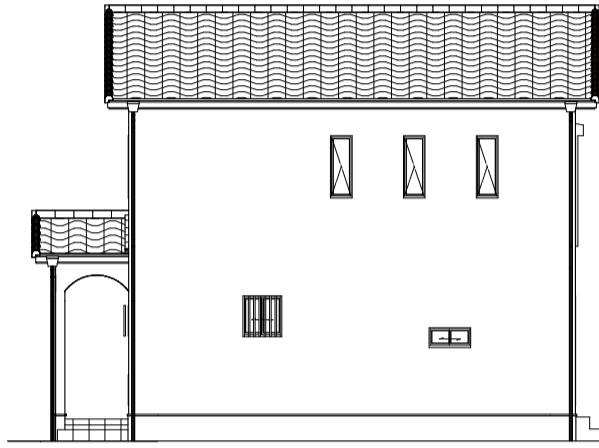
北側 立面図 S:1/100
