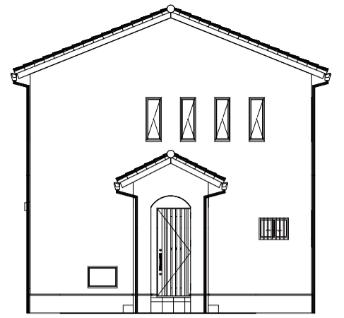
東側 立面図 S:1/100
