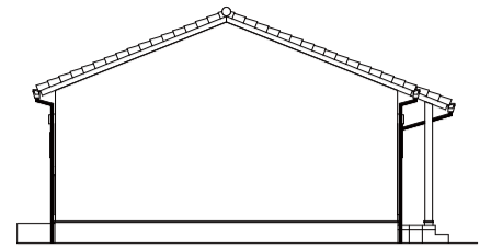
西側 立面図 S:1/100
