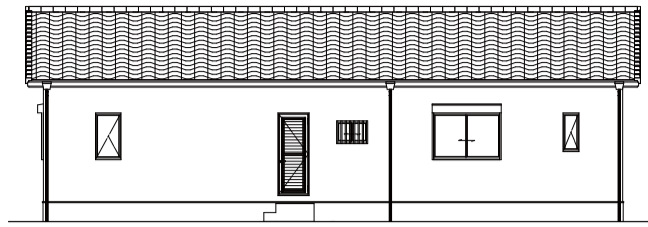
北側 立面図 S:1/100
