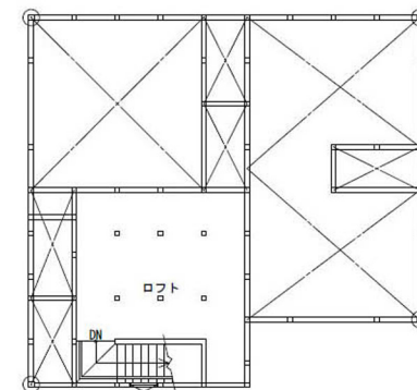
R階 平面図 S:1/100
