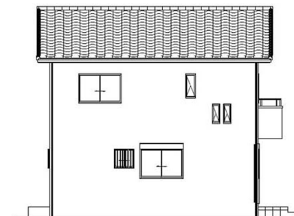
西側 立面図 S:1/100
