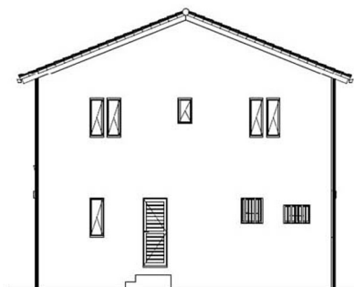
北側 立面図 S:1/100
