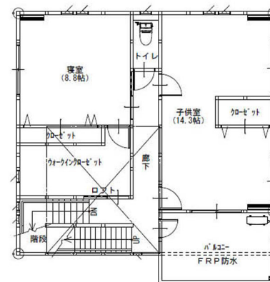
2階 平面図 S:1/100
