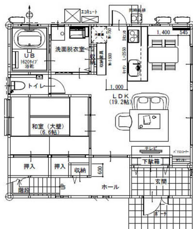
1階 平面図 S:1/100
